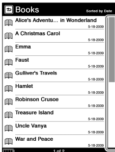
Scroll bar
